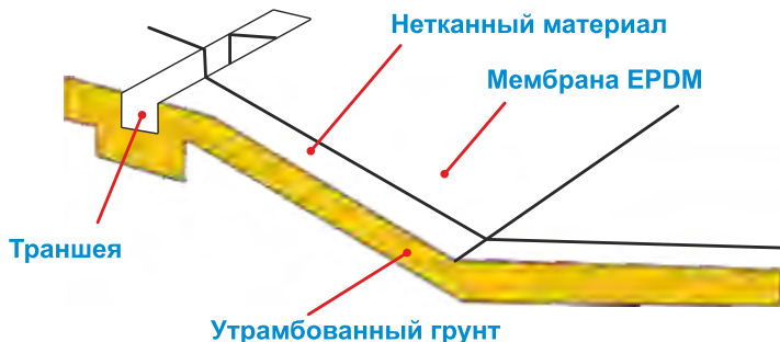
Рисунок 3. Схема организации пожарного водоема
